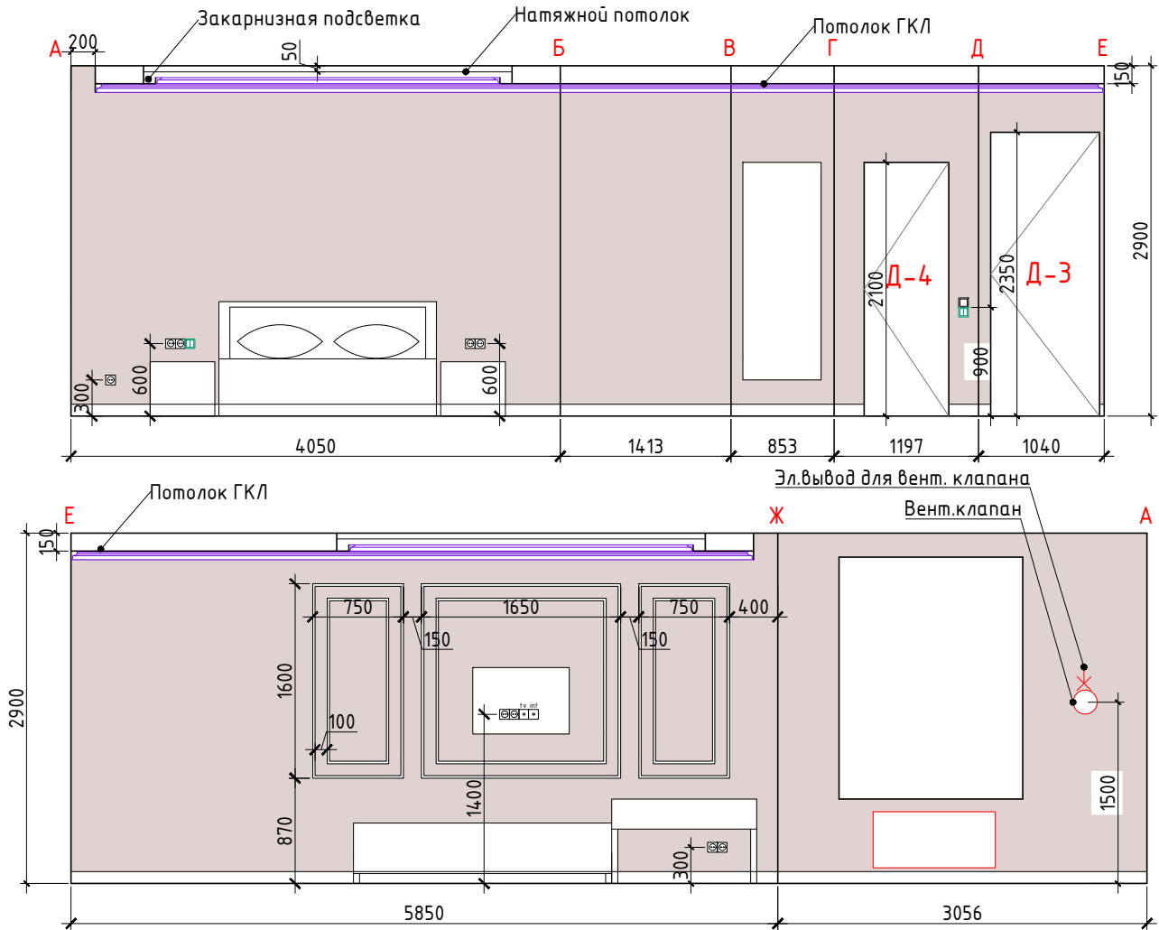
Гардеробная (помещение 4).
