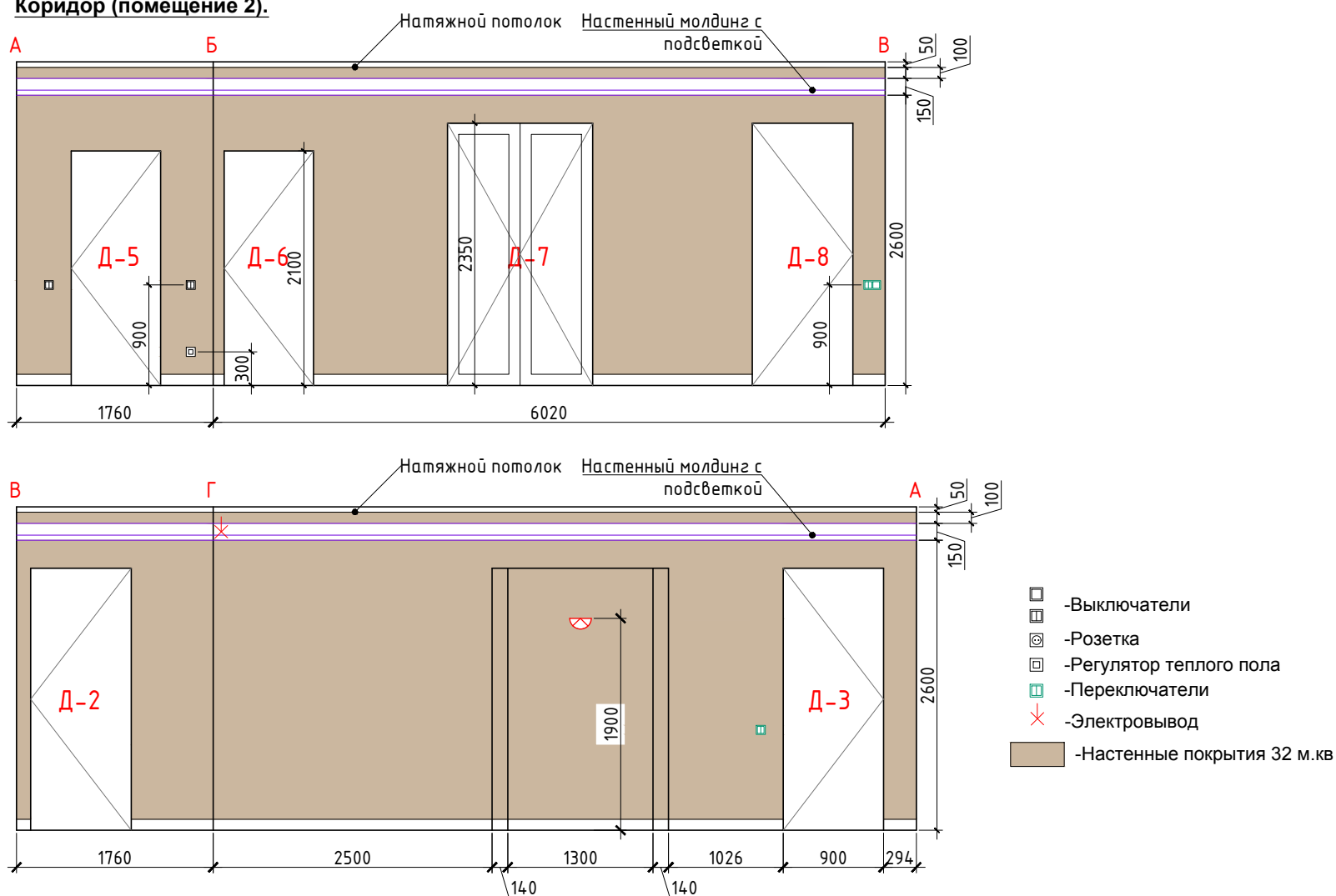
Коридор (помещение 2).
