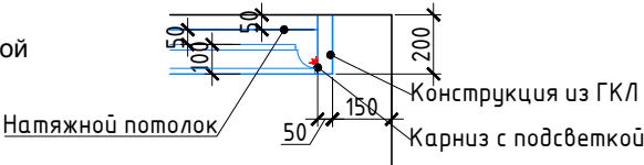
Разрез 2-2
